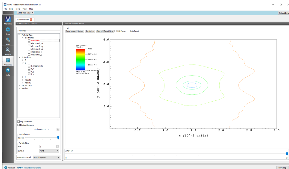
Fig. 11.12: Contours
