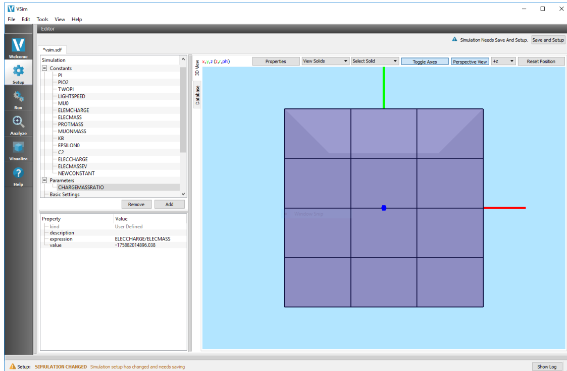
Fig. 6.4: Parameter definitions
